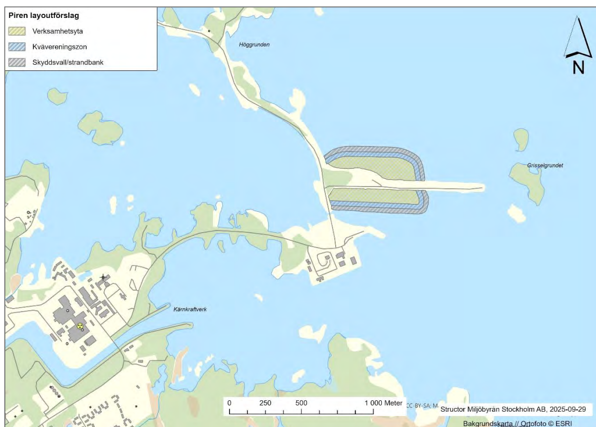
Figur 5-1. Layoutförslag för utfyllnad av piren.
