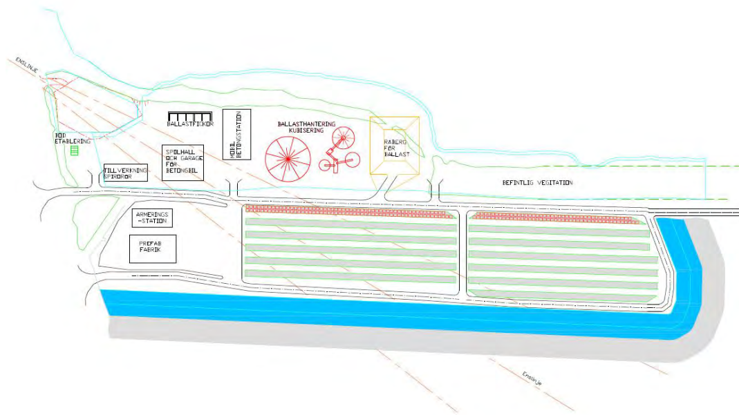
Figur 9-4. Verksamhetsyta då endast den södra delen av piren fylls ut. Betongstation och ballasthantering planeras på befintlig pir. Prefab-tillverkning och lagring av betongelement planeras på den utfyllda ytan under de inledande åren när pirens verksamhetsytor etablerats (cirka år 2027-2031).
