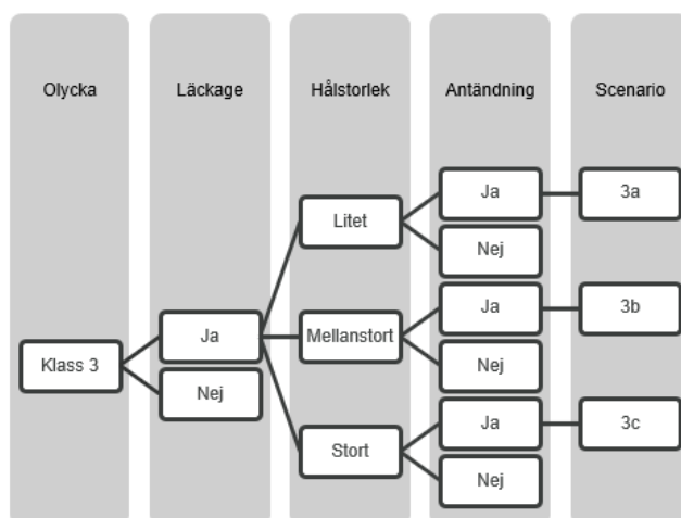
Figur 27 Händelsesträd för olyckor i farligt gods-klass 3.
