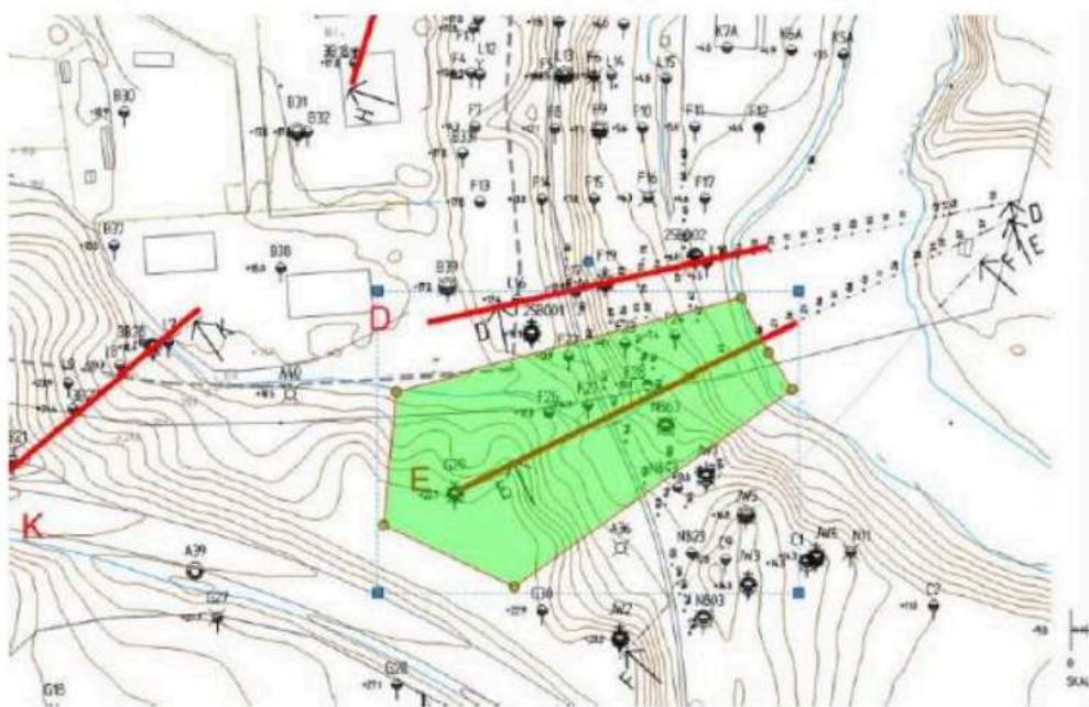
Figur 28. Område som behöver förstärkas (sektion E), enligt fördjupad geoteknisk utredning, daterad 2026-01-08.
