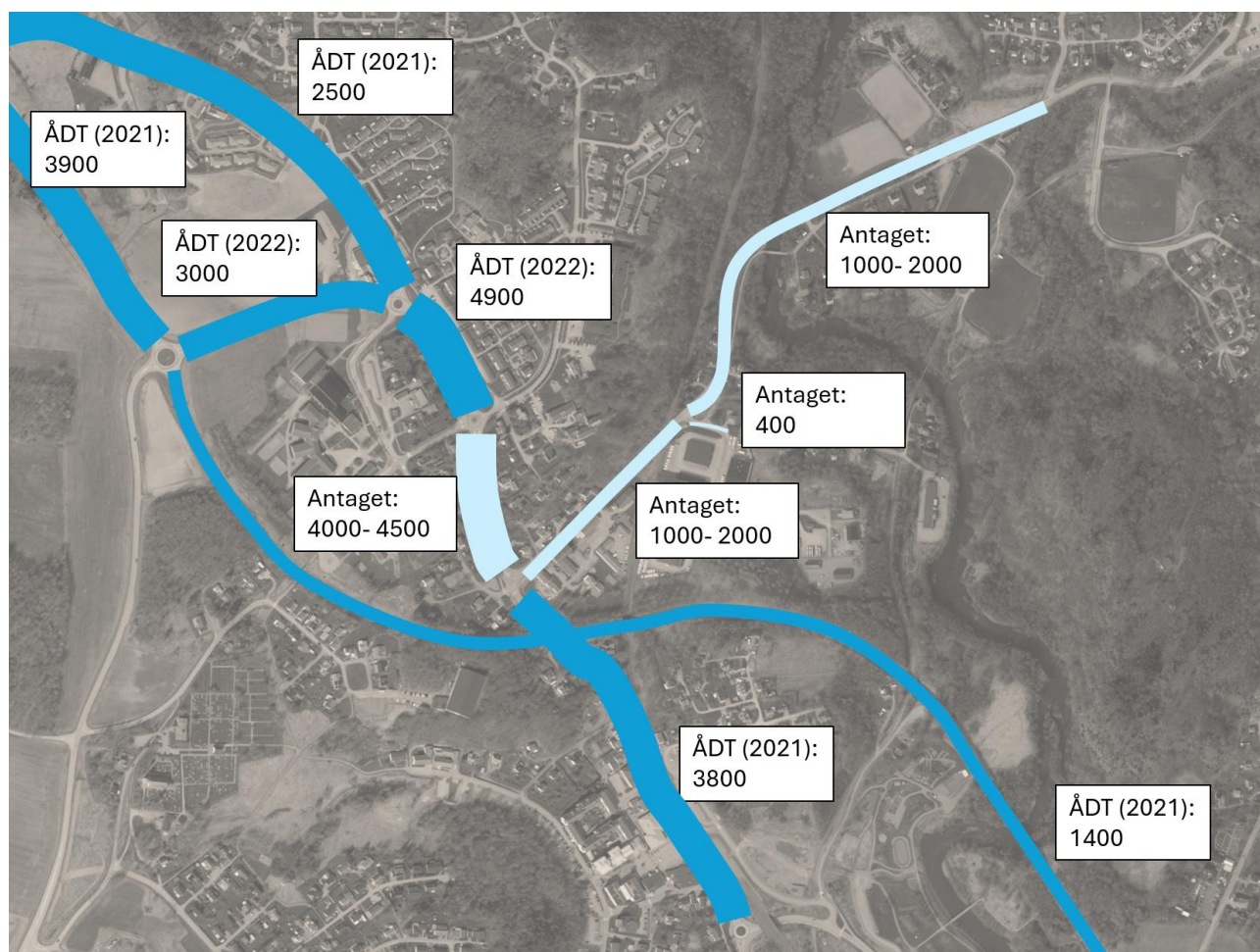
Figur 11. Uppmätta och antagna trafikflöden inom utredningsområdet i nuläget.
